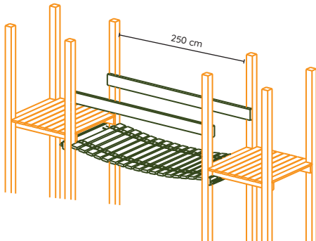
Pont de singe JT027
