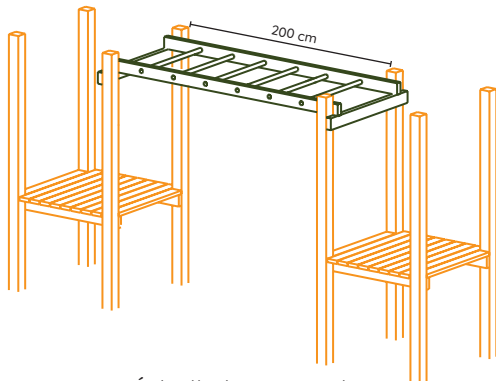
Échelle horizontale JT050
