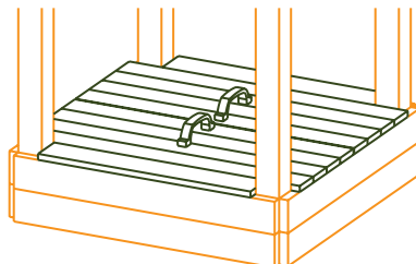
Couvercle bac à sable JT029
