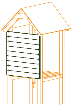
Fermeture JT024
