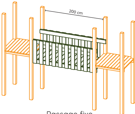
Passage fixe JT026
