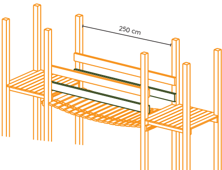
Mains courantes suppl. JT041
