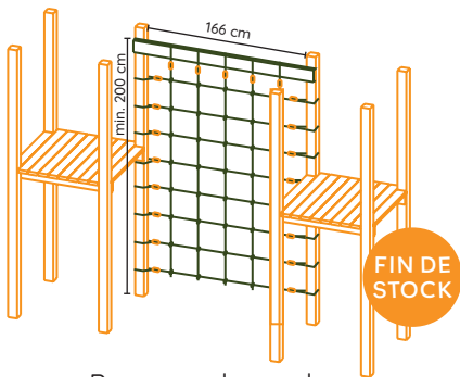
Passage de corde JT052
