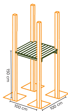
Plancher JT009
